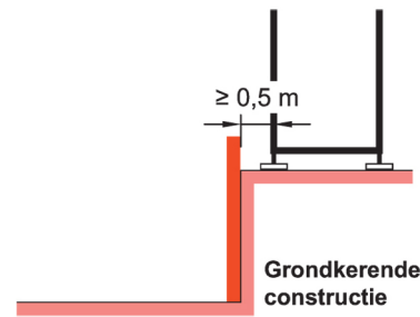
Grondkerende constructie
